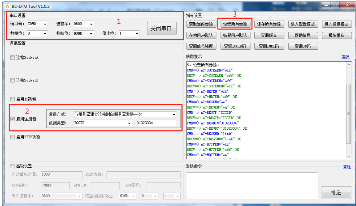
图 4-6 注册包参数设置
